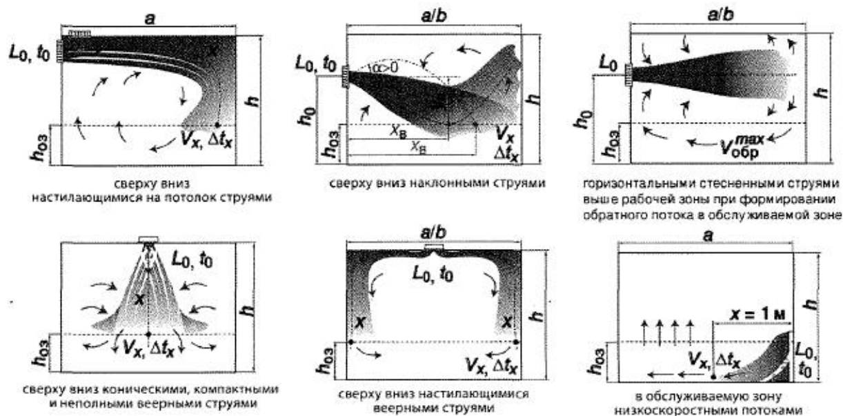
Рисунок Л.1 - Основные схемы подачи приточного воздуха
