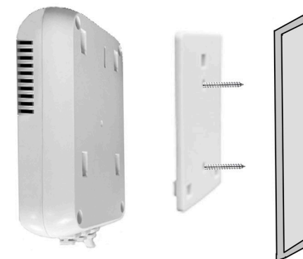
Прибор Крепежная пластина Стена
